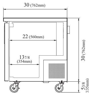
TUR-48SD-N-AL(-AR)
