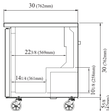
TUR-48SD-N
